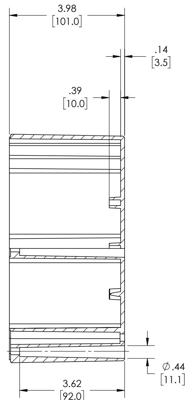
SECTION A-A
