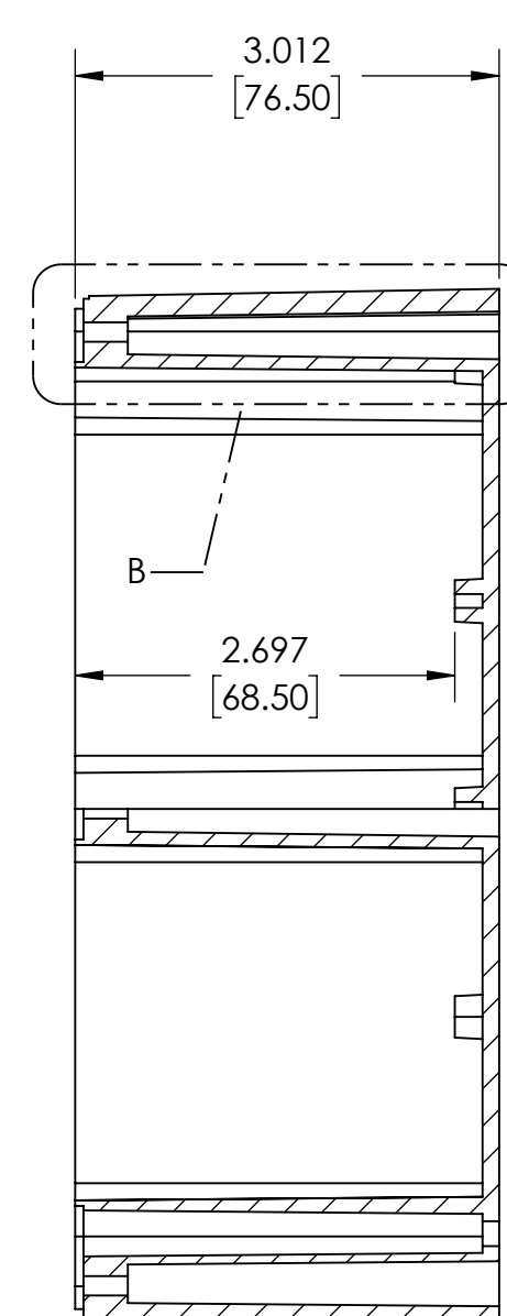
SECTION A-A
