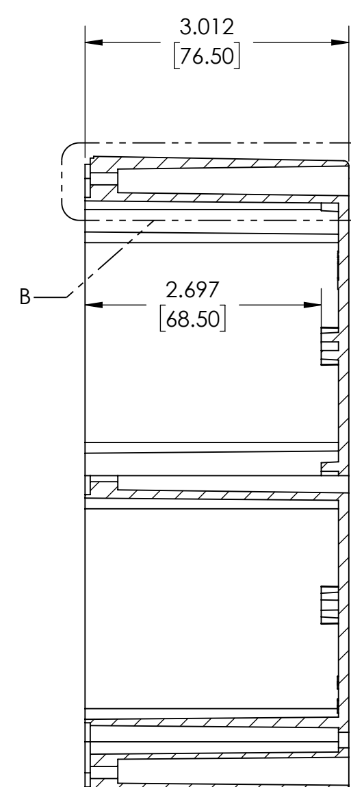
SECTION A-A
