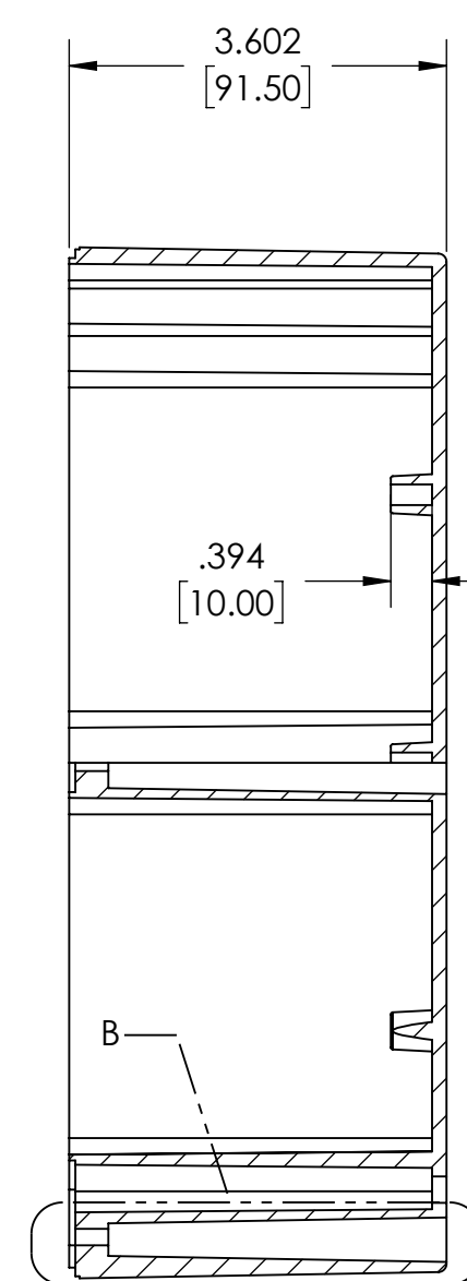
SECTION A-A
