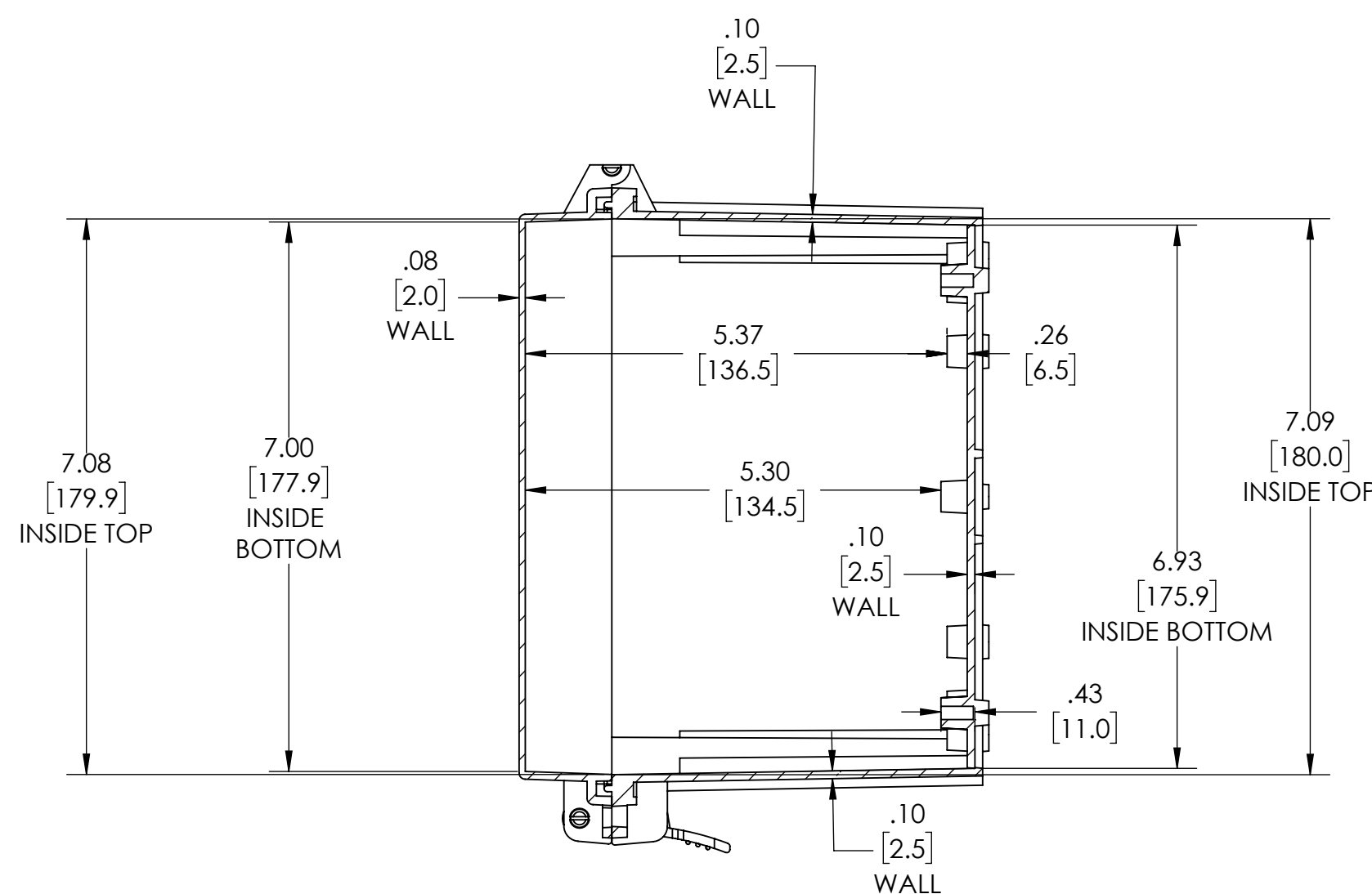
SECTION A-A
